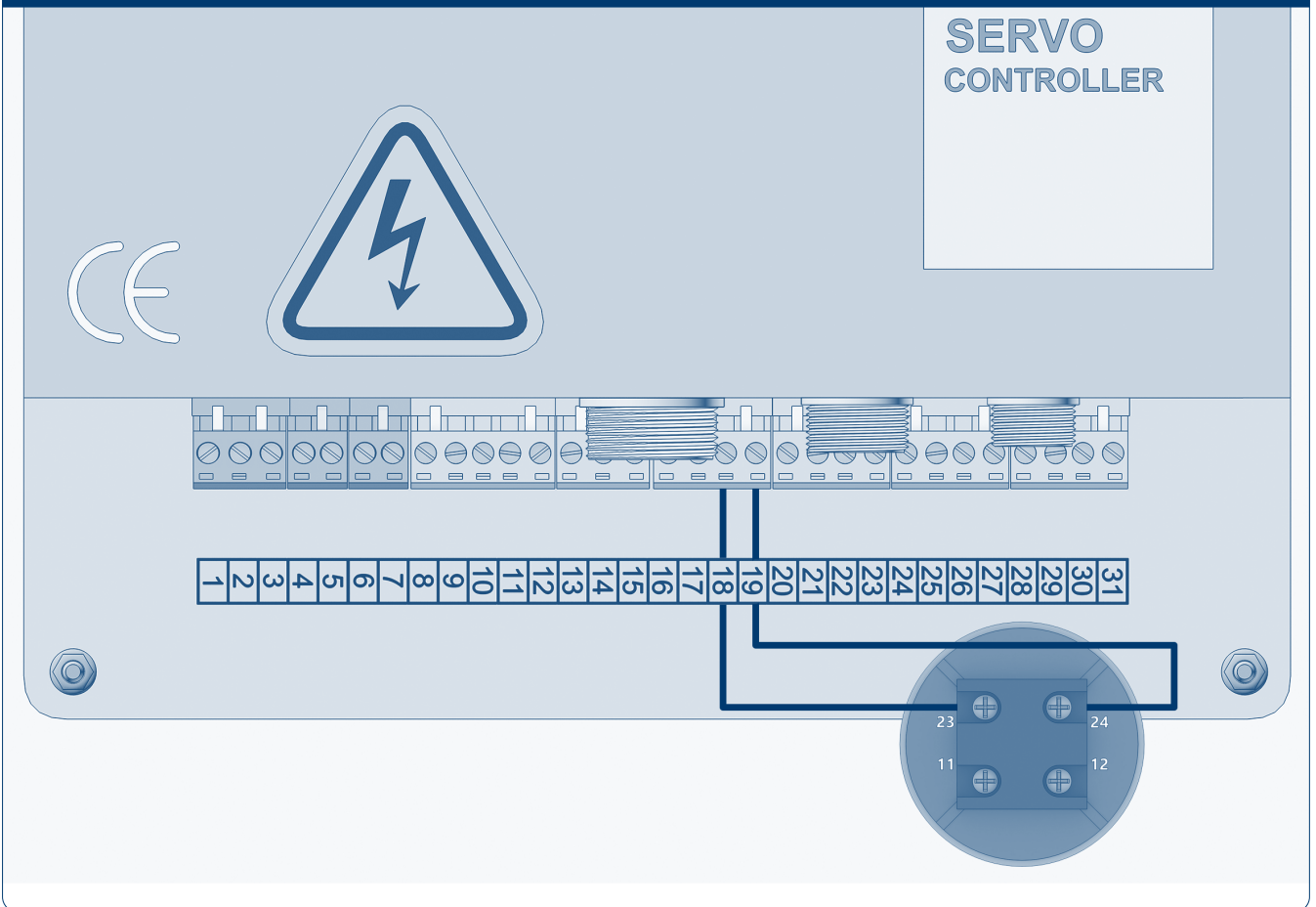
Рис. 14. Подключение кнопки, арт. DKH009, функция частичного открывания (0,75 кВт)
