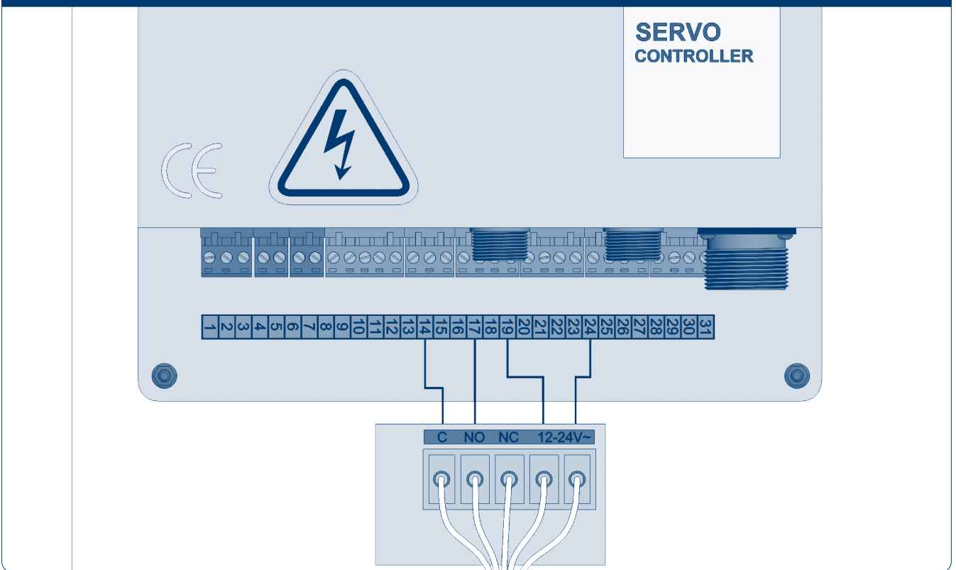
Рис. 15. Подключение радара, арт. HSD5007 (0,75 кВт)
