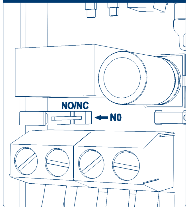
Рис. 40. Фотозлемент. Положение переключки — NO
